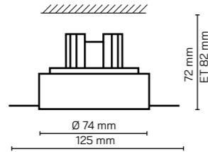
LED Einsatz 7W/10W
