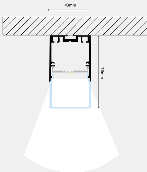
AUFBAU
